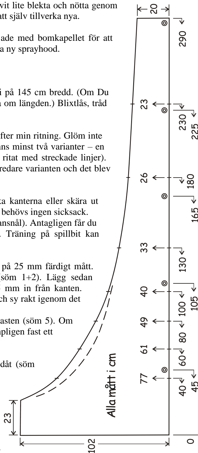
Bomkapell, Måtritning
